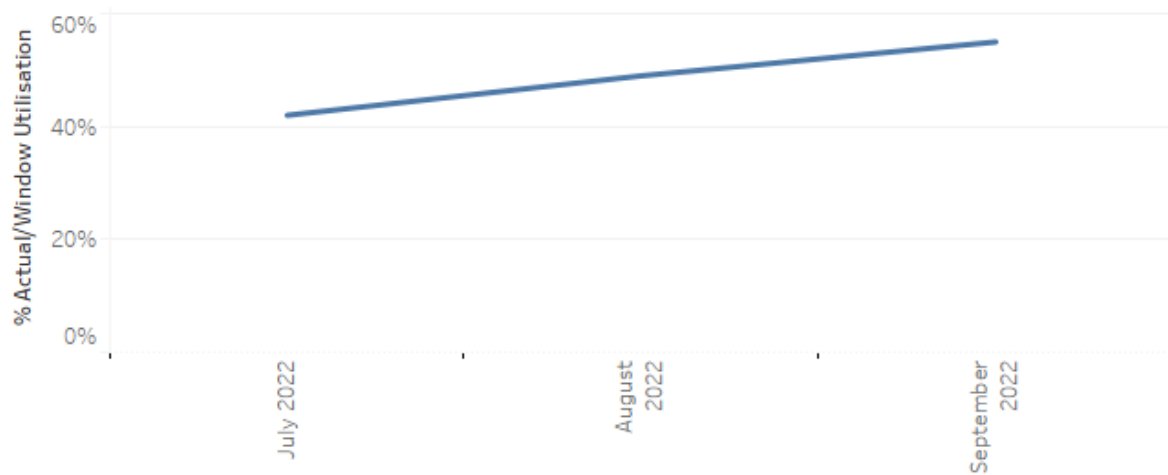
Port Botany Rail: % utilisation per month actual vs window (overall)
